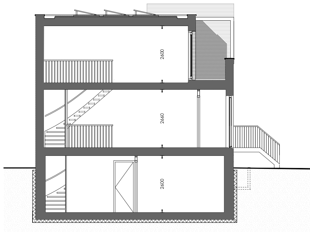
DOORSNEDE A-A
