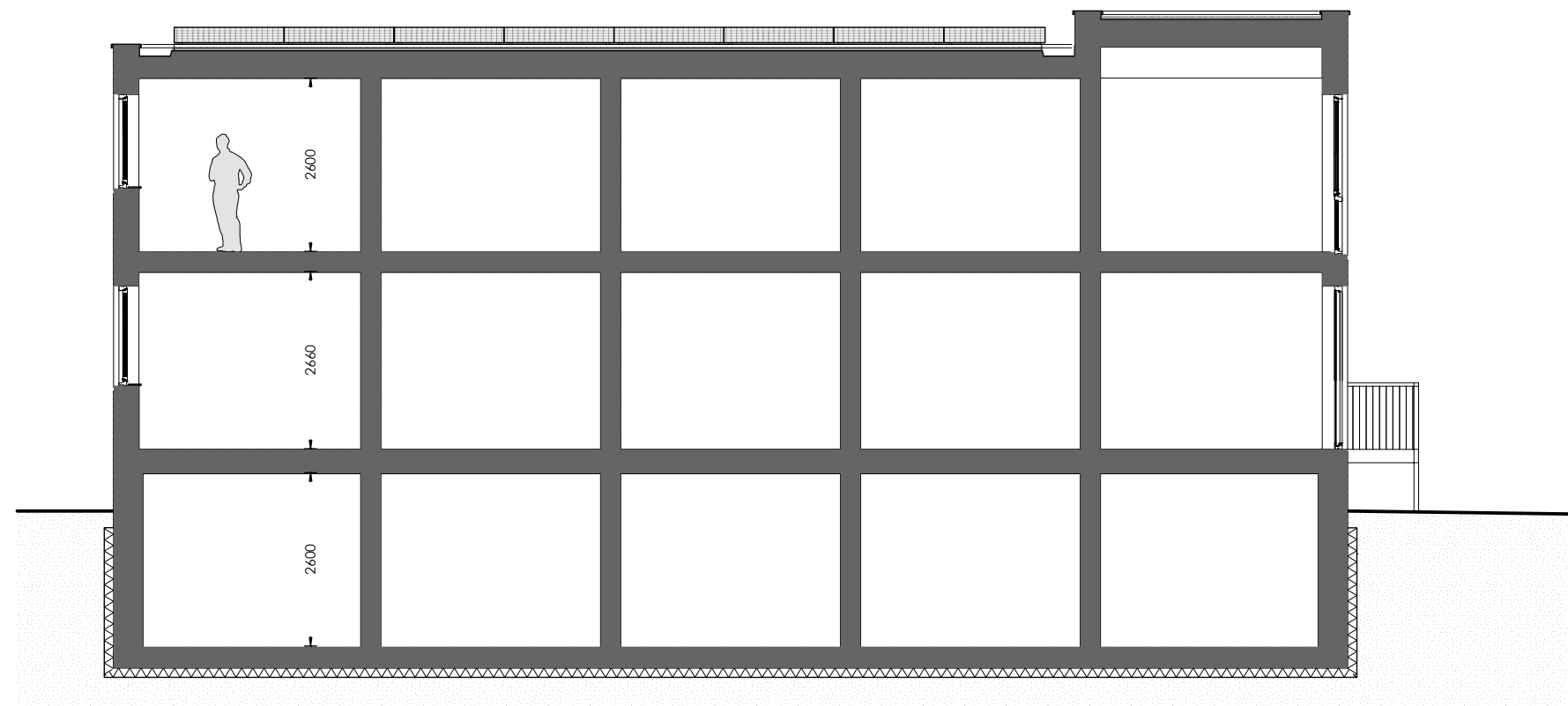
DOORSNEDE B-B
