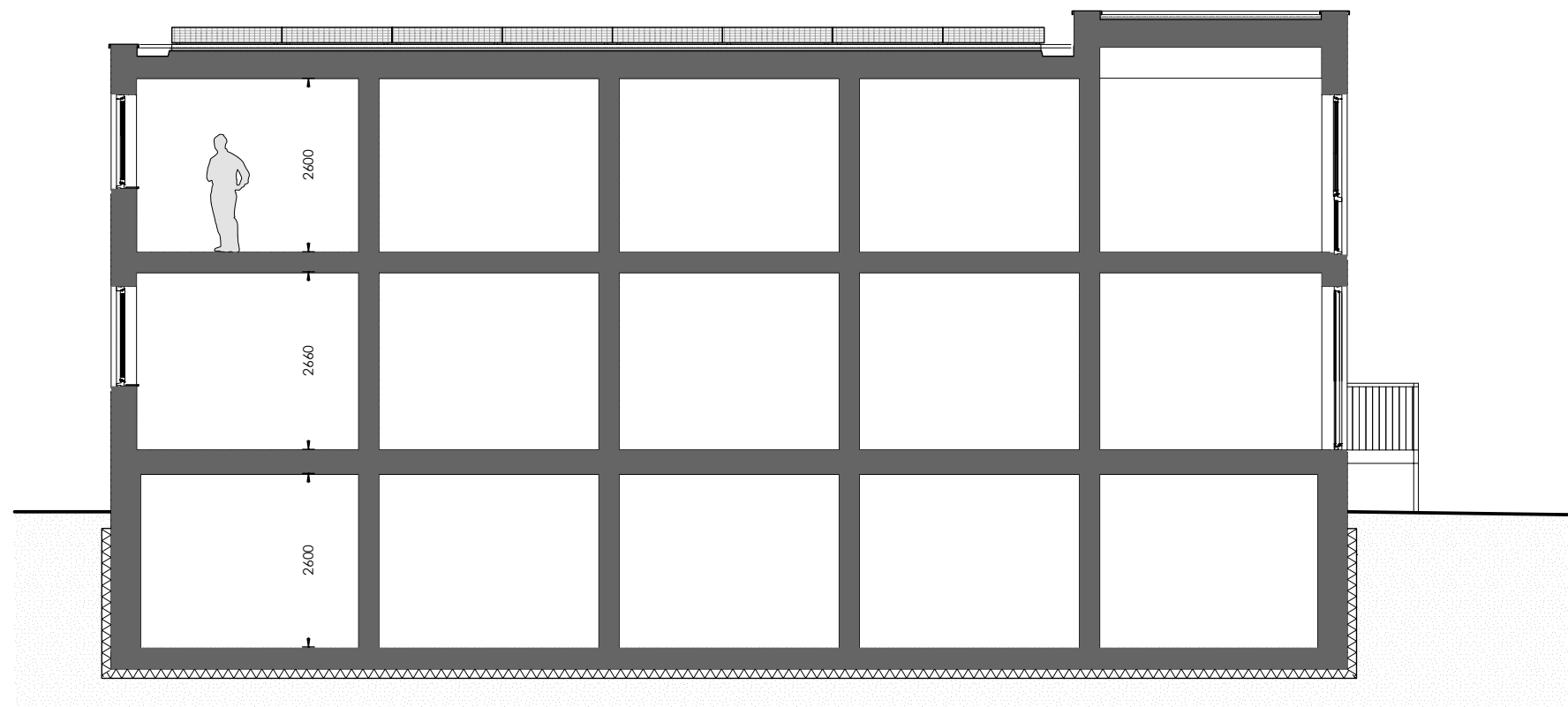
DOORSNEDE B-B
